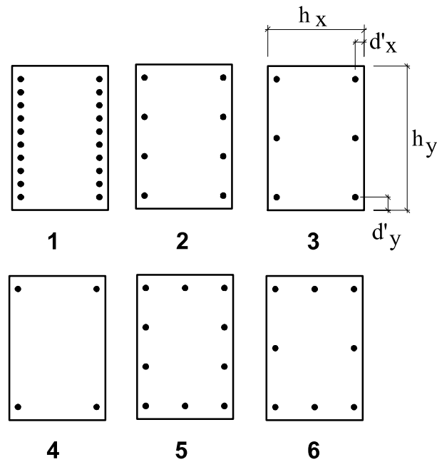
Figura 5 - Arranjos das barras
