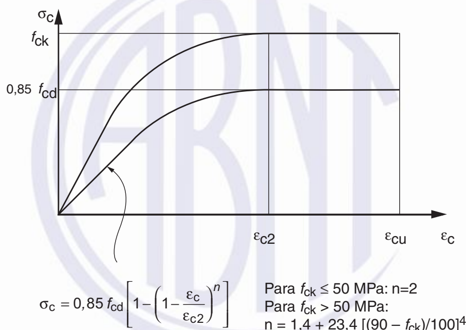
Figura 8.2 – Diagrama tensão-deformação idealizado
