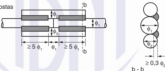
Figura 9.5 – Emendas por solda
