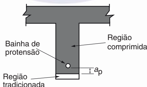
Figura 3.1 – Estado-limite de descompressão parcial
