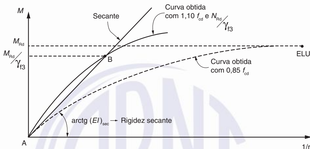
Figura 15.1 – Relação momento-curvatura
