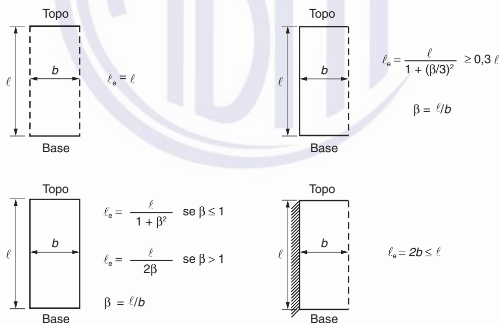
Figura 15.4 – Comprimento equivalente \ell_e
