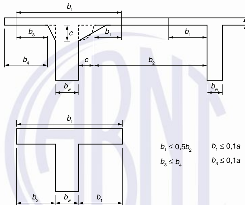
Figura 14.2 – Largura de mesa colaborante
