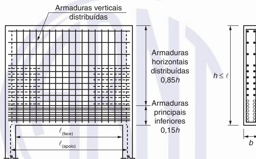
Figura 22.3 – Armação típica de viga-parede com h \leq l
