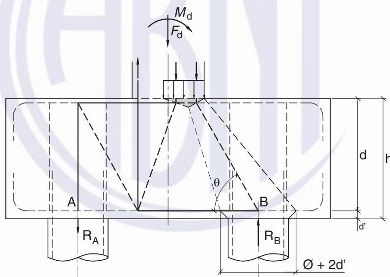
Figura 22.7 – Bloco com estacas tracionadas
