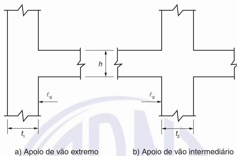
Figura 14.5 – Vão efetivo
