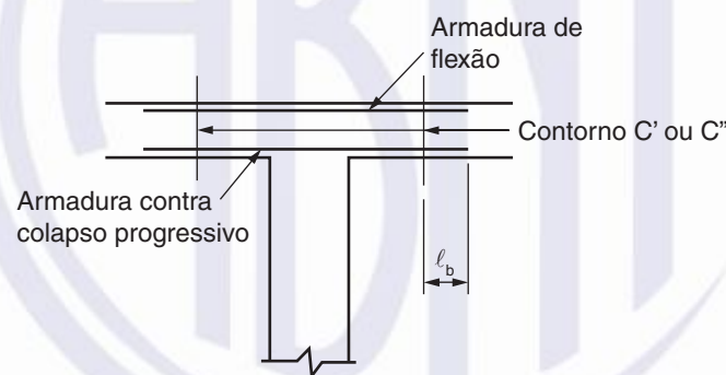
Figura 19.10 – Armadura contra colapso progressivo
